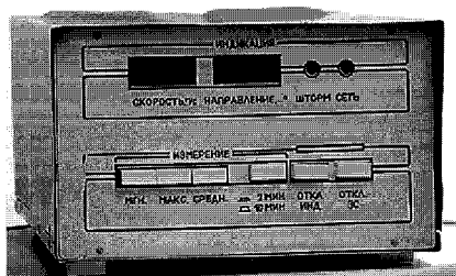
Сетевой анеморумбометр М-63. Блок датчиков скорости и направления ветра. Совместная работа ГГО, НИИ ГМП и Ленинградского завода «Гидрометприбор» в 1958—1960 гг. (Н. Г. Прокопцов, Д. Я. Суражский и А. Ф. Застенкер). а) датчик скорости и направления ветра, б) пульт анеморумбометра. Фото А. В. Цветкова.
