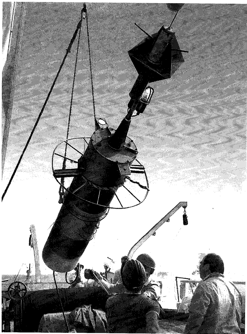
Дрейфующий буй, предназначенный для изучения подповерхностных течений.
