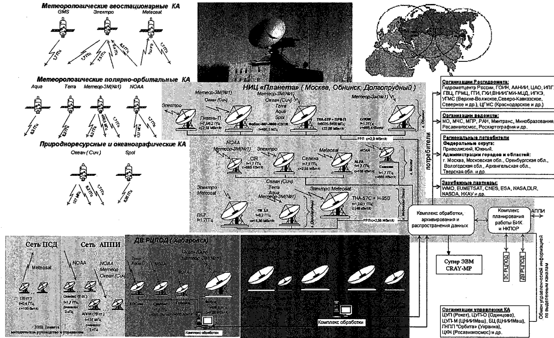
Рис. 2. Структурная схема наземного комплекса приема, обработки и распространения спутниковых данных (НКПОР Гидрометслужбы РФ).
