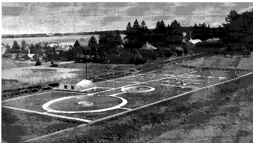
Водно-испарительная площадка Валдайского филиала Государственного гидрологического института.
