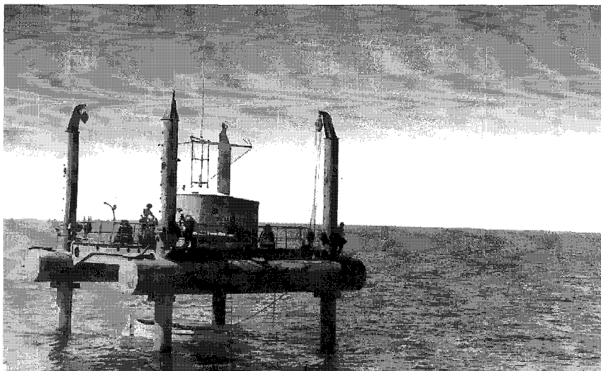
Свайное основание, установленное на Каспии для изучения характеристик моря.
