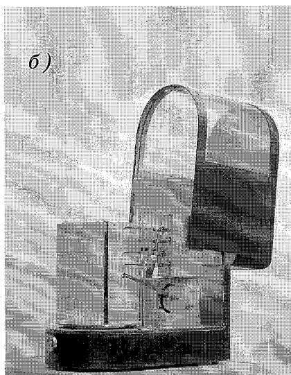
Электромеханический самописец ветра М-12 Разработан в ГГО (1954 г.), руководитель разработки — Н. Г. Протопопов. а) датчи скорости и направления ветра, б) регистратор Фото А. В. Цветкова.
