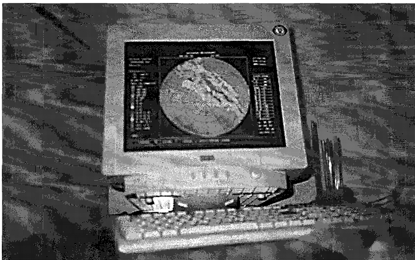
Радиоэхо облаков и осадков фронта окклюзии. МРЛ-5, масштаб развертки 200 км. ИКО
